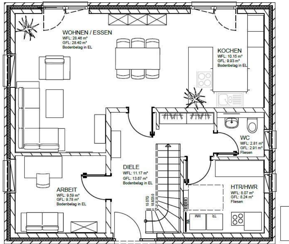
Erdgeschoss
