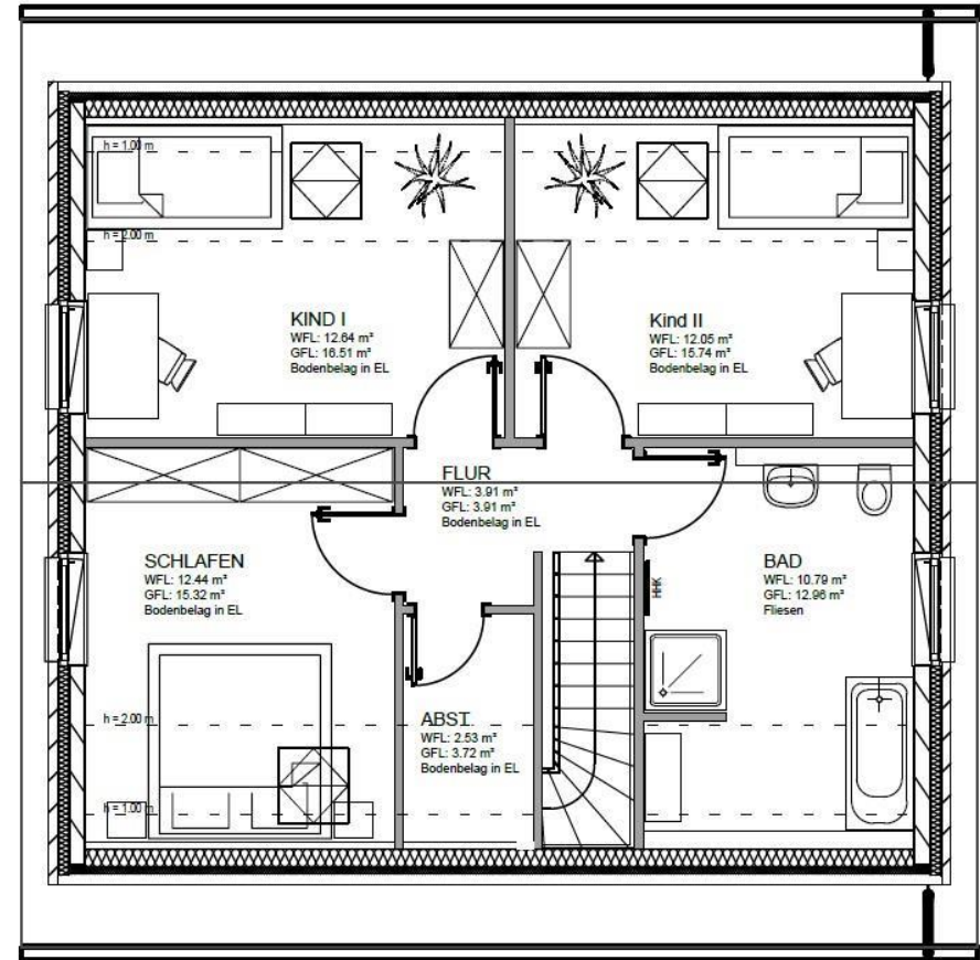
Dachgeschoss
